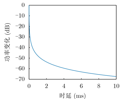
图4 多径信道模型归一化时延-功率谱
