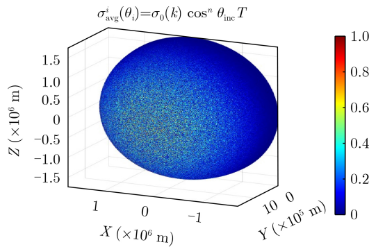
图2 月球表面RCS近似分布
