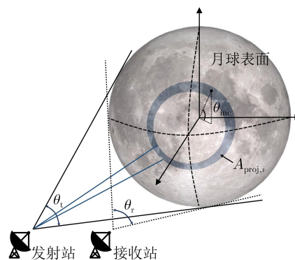
图1 统一积分模型反射场景示意图
