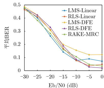
图5 不同均衡策略在多径信道模型下的性能
