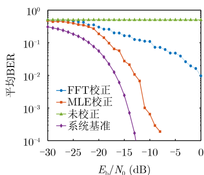
图6 不同信噪比下的误码率(10 kHz频偏)
