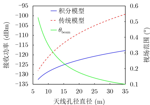
图3 积分模型接收功率vs传统模型接收功率
