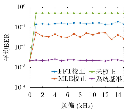
图7 不同频偏下的误码率(SNR=-15 dB)
